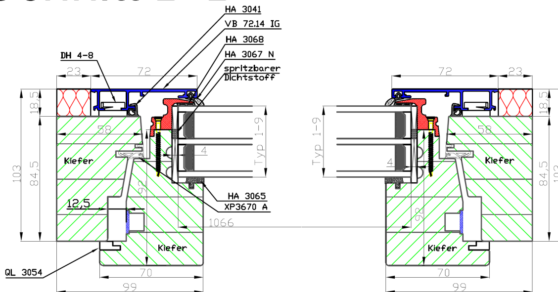
Bild 4 Horizontalschnitt, geprüft wurde mit 8/18/4/18/6 Verglasung (Typ 3)
